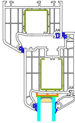
BB - DETAYI
