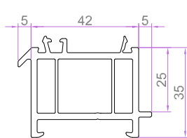
KÖRKASA YÜKSELTME 7257 0.658 kg/m
