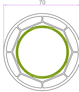
KÖŞE DÖNÜŞ BORUSU 7254 1.044 kg/m
